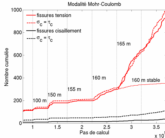
Figure 6. Nombre cumulée de microfissures dans l'inclusion PFC2D à différents étapes de la vidange (lignes verticales). L'étape à 160 m a été prolongée pour trouver la stabilité. Une claire instabilité est notée à partir de 165 m.
