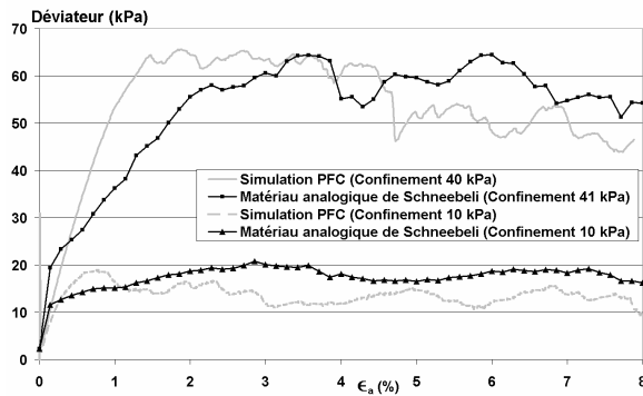
Figure 2 : Courbes de contrainte déviatorique-déformation axiale (matériau frottant).
