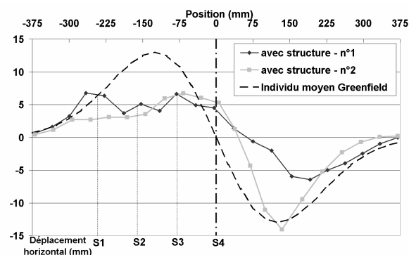
Figure 6 : Déplacement horizontal avec structure (modèle réduit physique). Figure 7 : Déplacement horizontal avec structure (modèle numérique).
