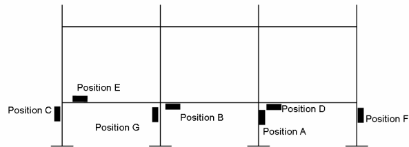
Figure 8 : Position des jauges sur la structure.
